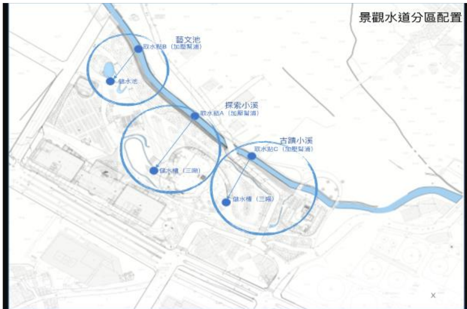
圖 4-17 隆恩圳千甲段景觀小溪分區配置圖
